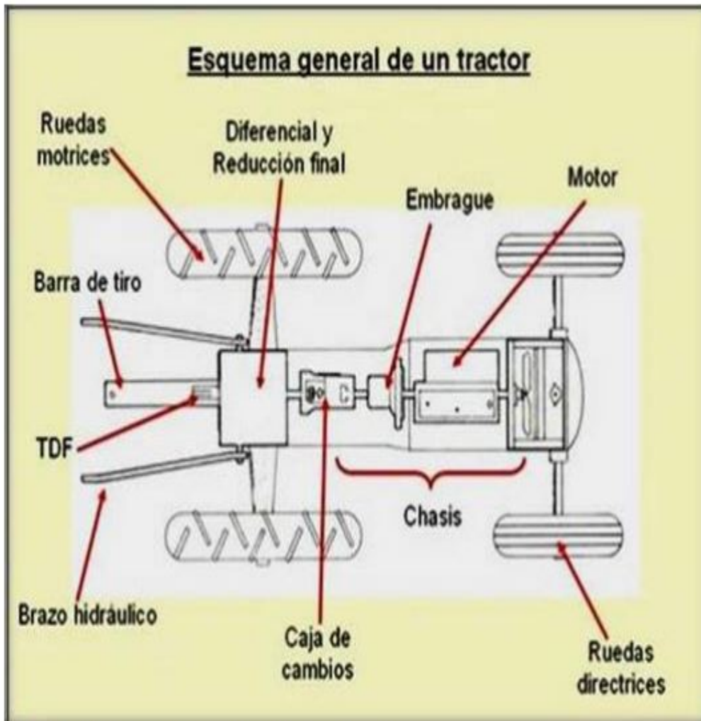
Figura 1. Componentes principales de un tractor.
